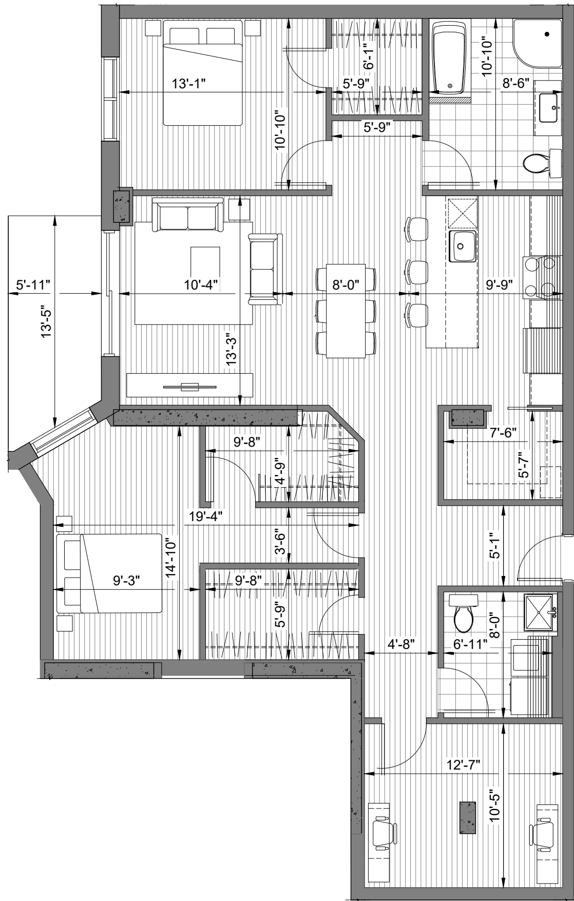
E UNITÉ 5 1/2 ECHELLE: 1:75
